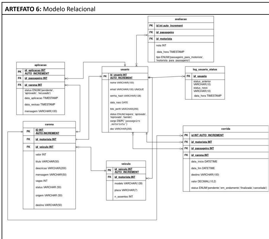
Figura 6 – Modelo Relacional (DRAW.IO)
